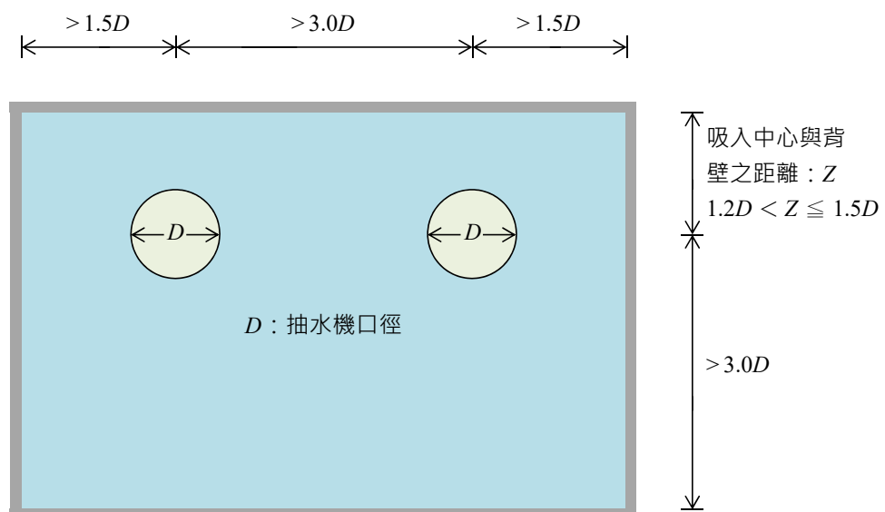
圖 6-1 抽水井配置尺寸示意圖
