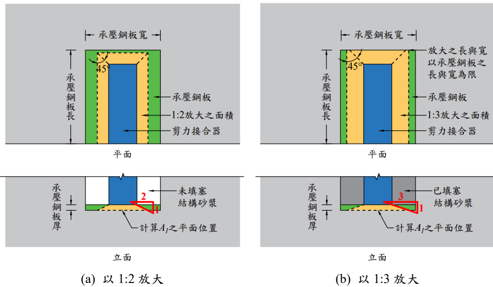
圖 R8.4 承載面積 A_1 之計算方式
