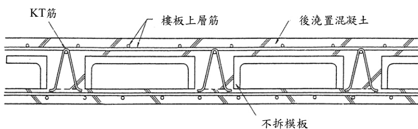
圖 R7.27 中空合成樓板例 [7.5]
