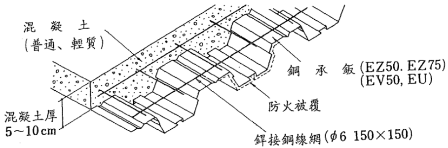
圖 R7.22 鋼承板合成樓板例(單位：mm) [7.5]
