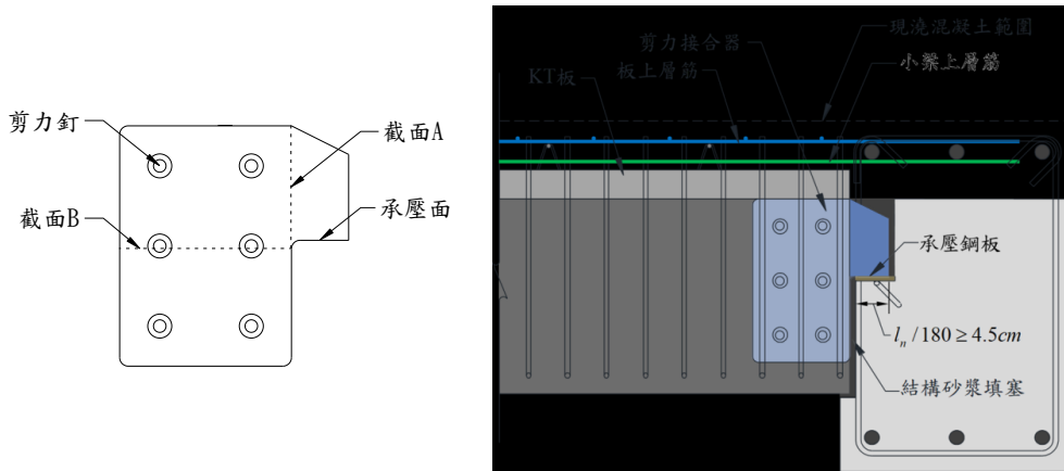
(a) 剪力接合器示意圖
