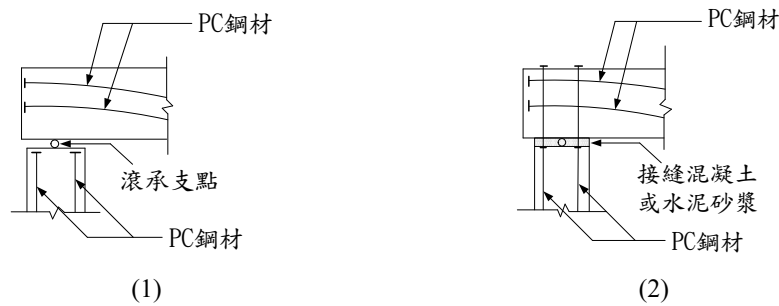
圖 R7.19 不產生二次應力之接合法例 [7.5]
