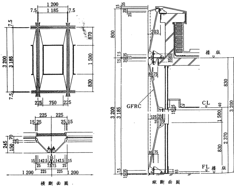
圖 R7.37 GFRP 帷幕牆圖例(單位：mm) [7.5]
