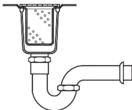
圖4-22 毛髮截留器參考圖例
