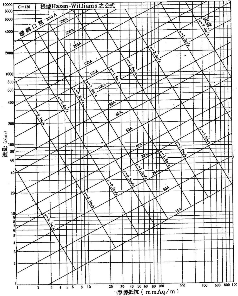
圖 A-7 內襯 PVC 鋼管摩擦抵抗線圖
