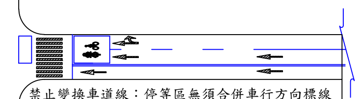
停等區合併標線示意圖
