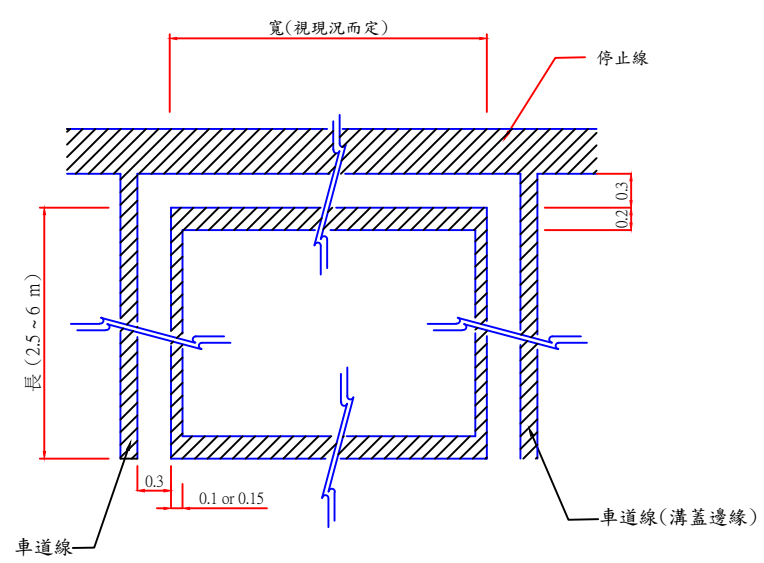
34 機慢車停等區線§174-2 (寬x2x0.2+長x2x0.1~0.15)
