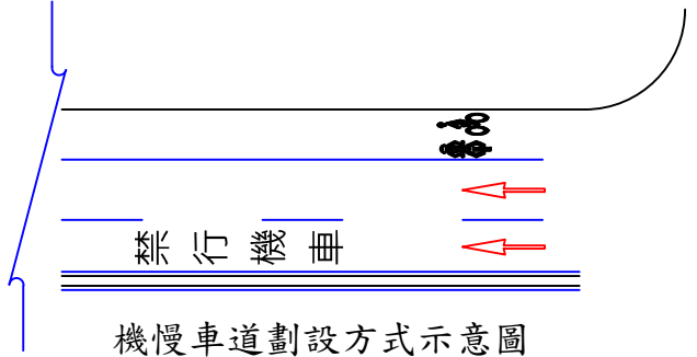
機慢車停等區劃設方式示意圖
