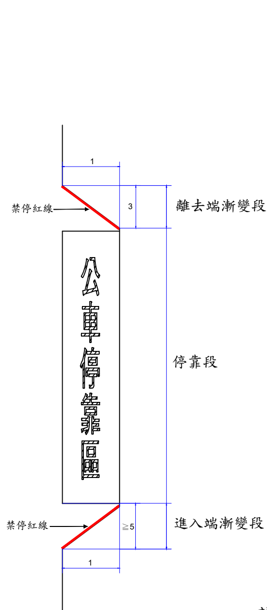
公車彎劃設圖例
