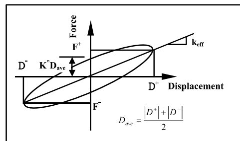
圖 C10-6 固態黏彈性元件之理想化受力變形關係
