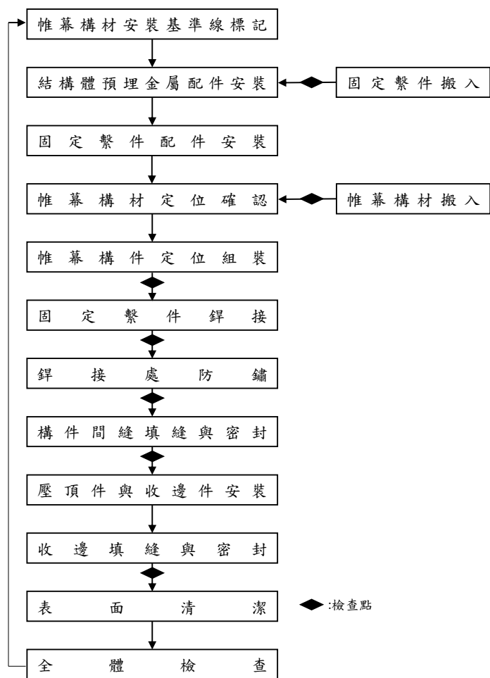
圖 R7.2 帷幕預鑄混凝土工法安裝組立流程例
