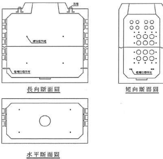
圖 3.4-5 纜線管路手孔示意圖
