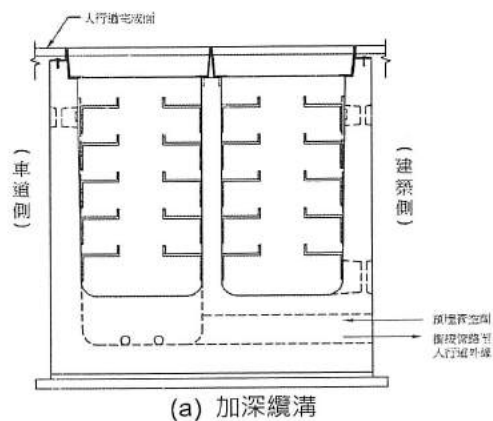
圖 4.4-2 電纜溝電纜分匯部構造示意圖
