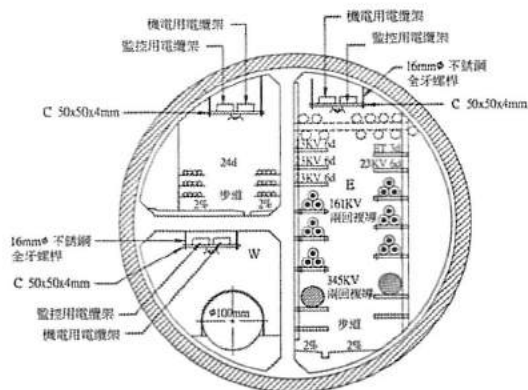
圖 3.4-1 箱型共同管道斷面配置示意圖
