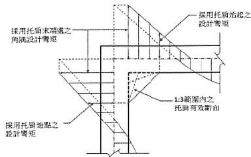
圖 4.1-2 角隅之設計彎矩圖
