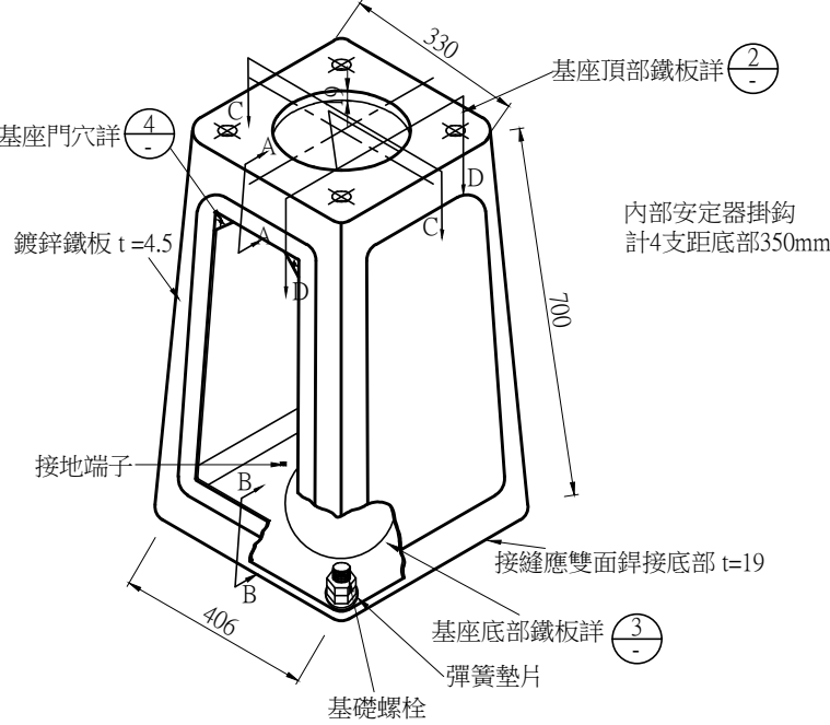
H型基座式分電箱詳細圖 NTS Unit:mm
