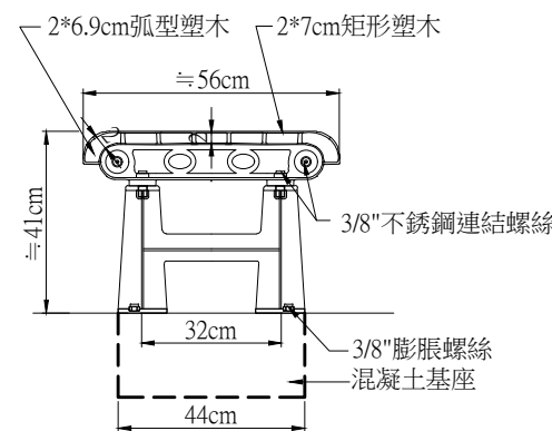
側立面圖
