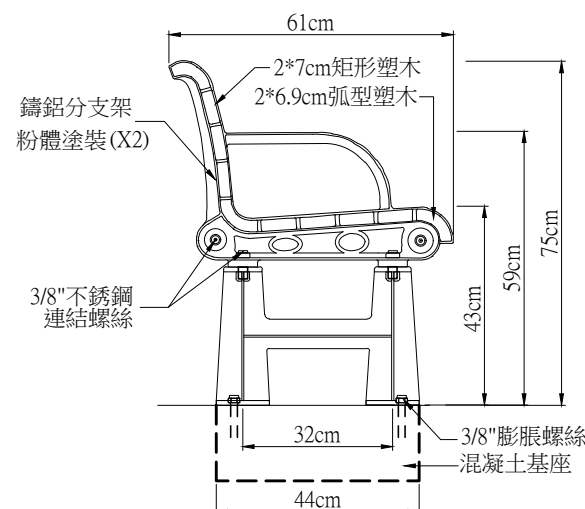
側立面圖
