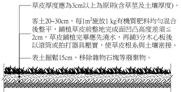
草皮種植(客土回填)示意圖 NTS Unit:cm
