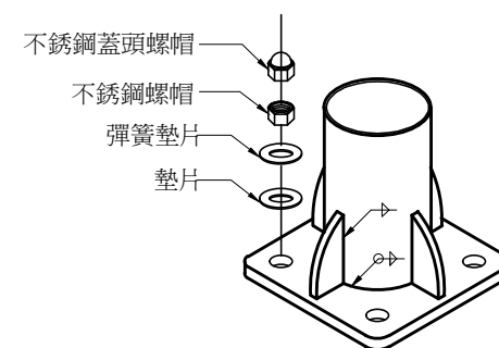
燈桿底板組合示意圖 NTS Unit:mm 4 -
