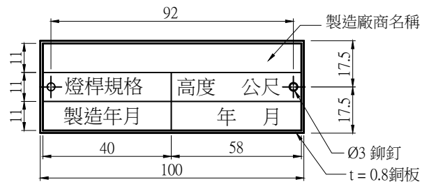
製造廠商名牌詳圖 A1 (1:1) A3 (1:2) Unit:mm 本名牌字體以凸字顯示 3
