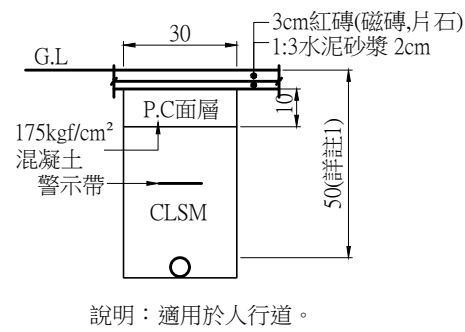
說明：適用於人行道。 DUCT D1(人工) NTS Unit:cm
