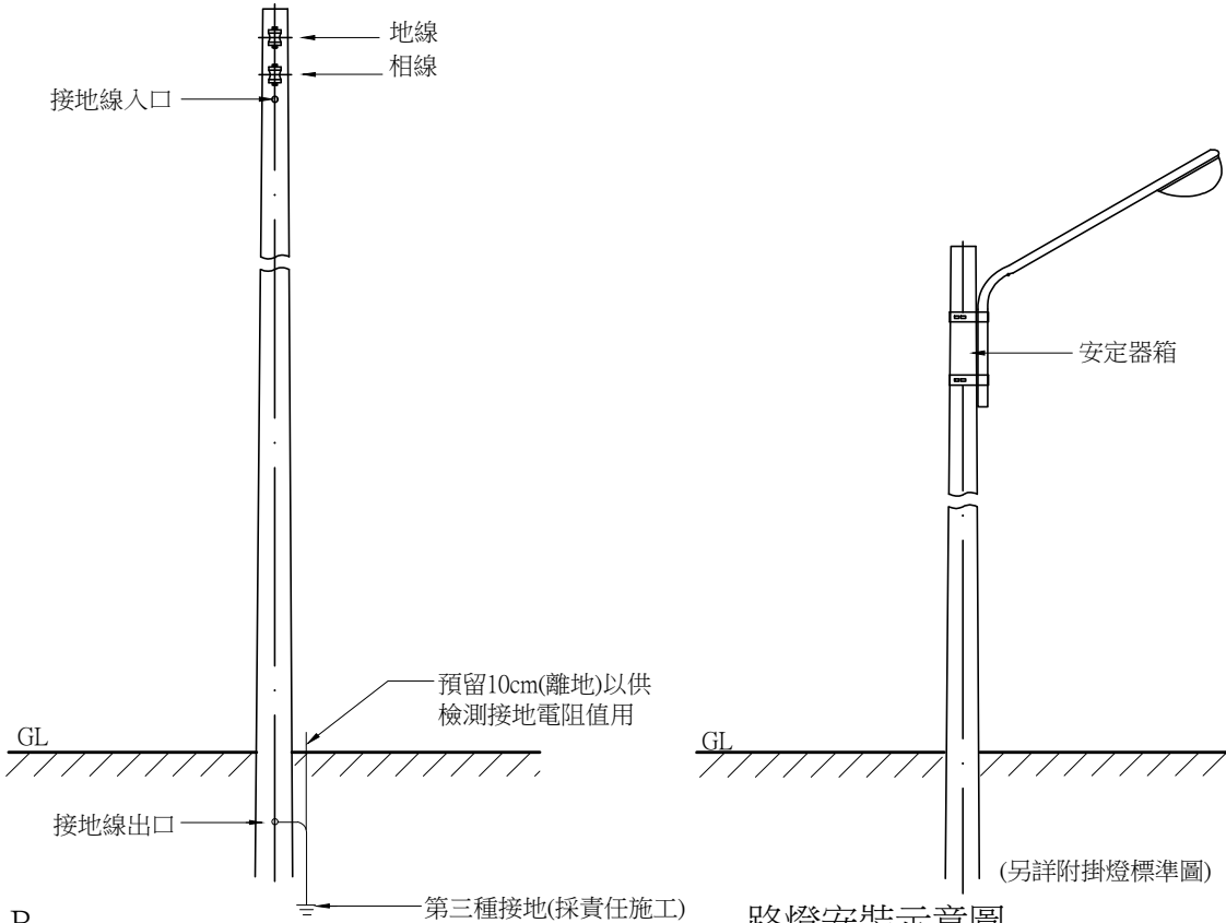
安裝圖 B NTS Unit:mm =2
