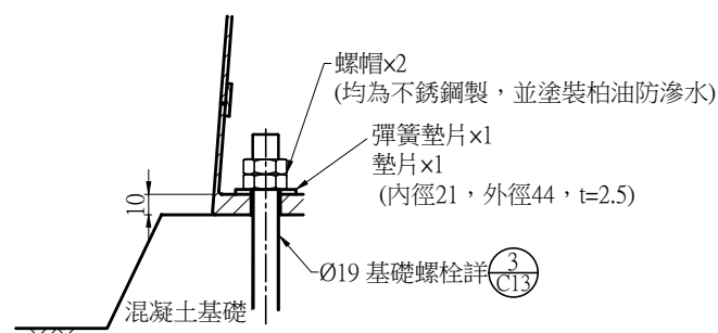
L 型基座 B-B 詳圖 A1 (4:1) A3 (2:1) Unit:mm
