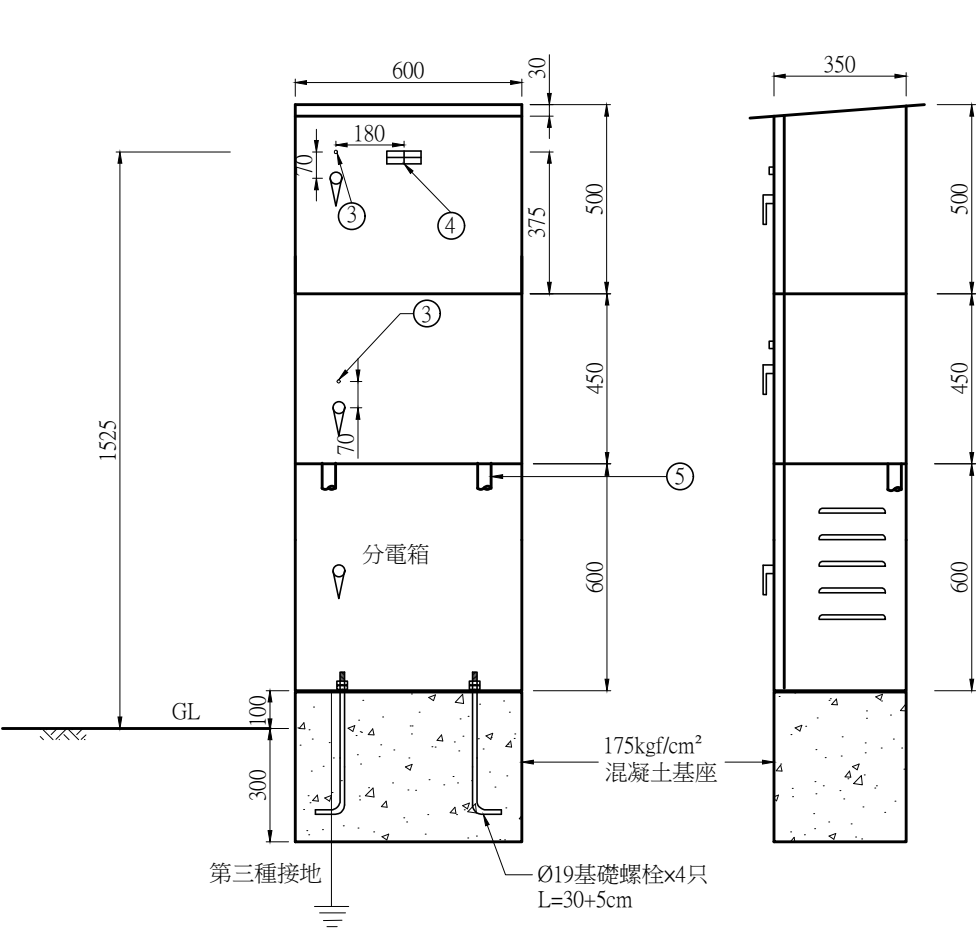
電表箱詳圖
