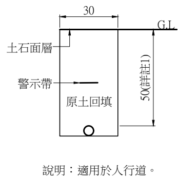
說明：適用於人行道。 DUCT B1(機械) DUCT B2(人工) NTS Unit:cm
