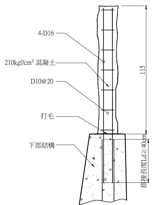
剖面圖 A1 (1:10) A3 (1:20) Unit:cm
