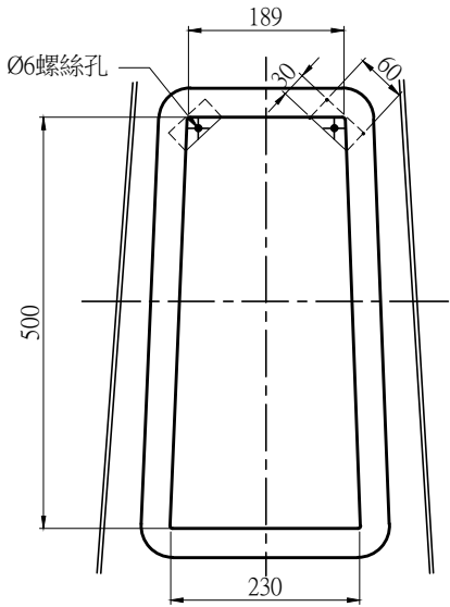
H型基座門穴詳圖 A1 (1:5) A3 (1:10) Unit:mm
