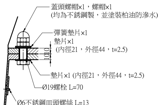
L 型基座 A-A 詳圖 A1 (4:1) A3 (2:1) Unit:mm
