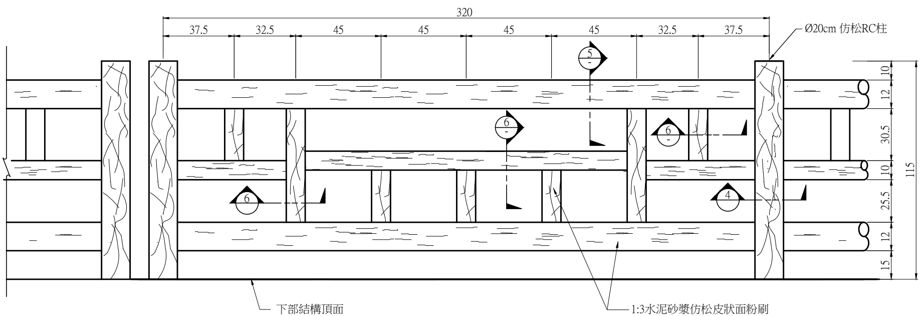
仿松欄杆(TYPE II)立面圖 A1 (1:10) A3 (1:20) Unit:cm
