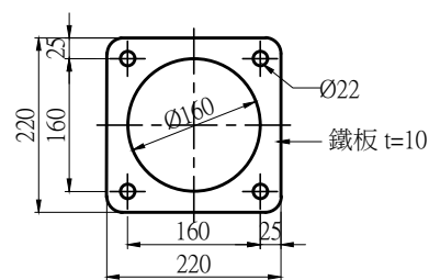
L 型基座頂部鐵板詳圖 A1 (1:5) A3 (1:10) Unit:mm
