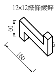
腳踏釘組詳圖 NTS Unit:mm 2 -
