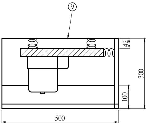
內部頂視圖
