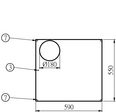
中間隔板
