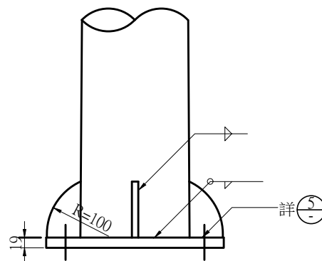
燈桿底板詳圖 NTS Unit:mm
