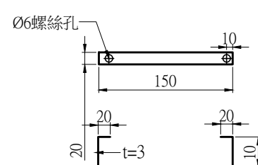
L 型基座底部鐵板詳圖 A1 (1:3) A3 (1:6) Unit:mm
