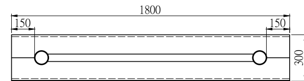
槽鋼護欄平面圖 NTS Unit:mm
