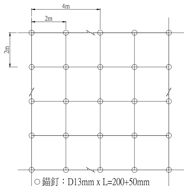
錨釘平面圖 NTS Unit:m
