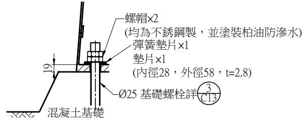
H型基座B-B 詳圖 A1 (1:1) A3 (1:2) Unit:mm
