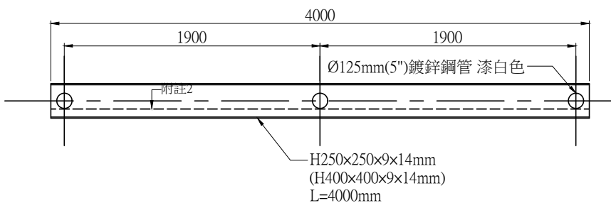
型鋼護欄平面圖(4m) NTS Unit:mm
