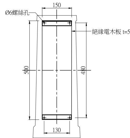
L 型基座 C-C 詳圖 A1 (1:5) A3 (1:10) Unit:mm
