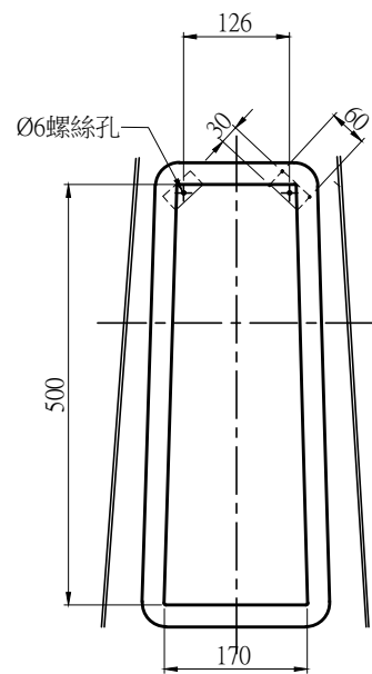
L 型基座門穴詳圖 A1 (1:5) A3 (1:10) Unit:mm
