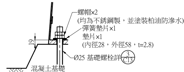
H型基座底板剖面圖
