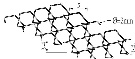
立體網示意圖 NTS Unit:cm
