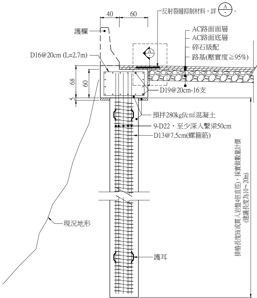
排樁詳圖(樁徑Ø=60cm)
