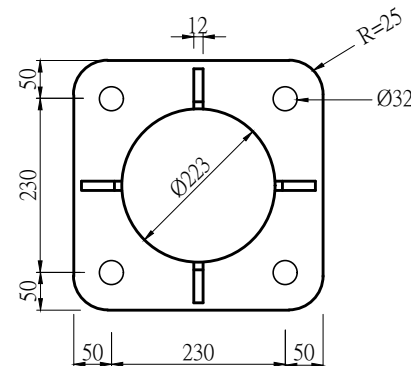
燈桿底板詳圖 NTS Unit:mm
