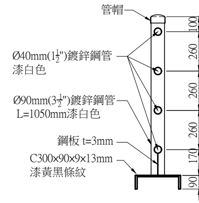
槽鋼護欄剖面圖 NTS Unit:mm
