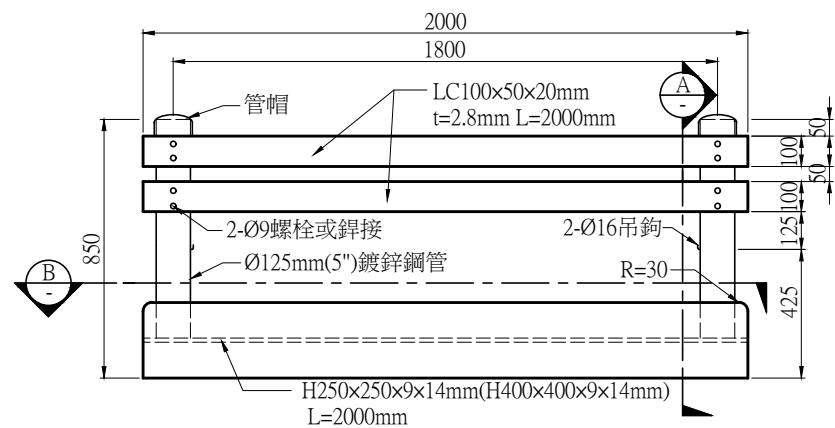
型鋼護欄正立面圖(2m) NTS Unit:mm
