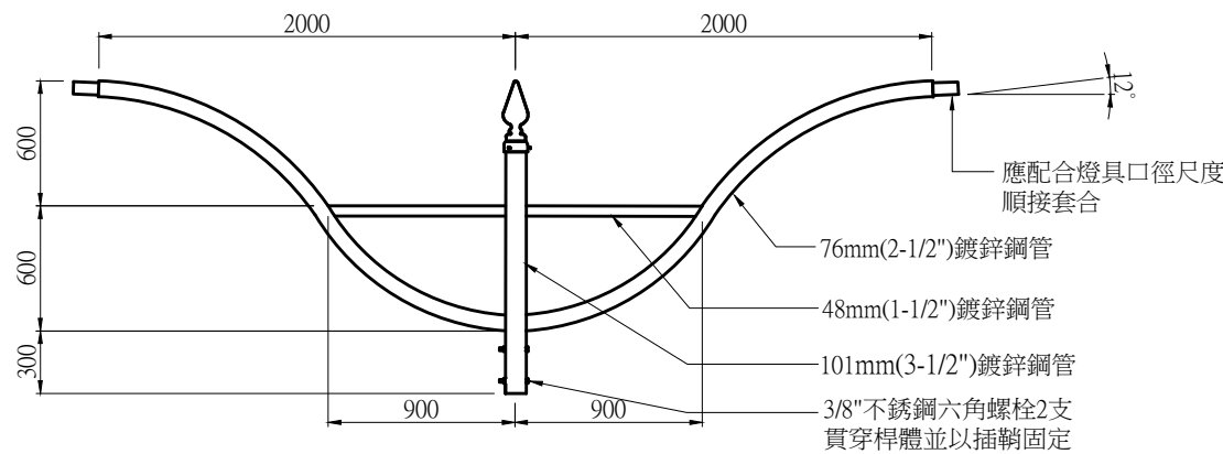
活動式燈架詳圖 NTS Unit:mm
