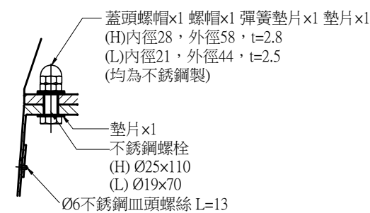
底板、基座接合詳圖 NTS Unit:mm 5 -
