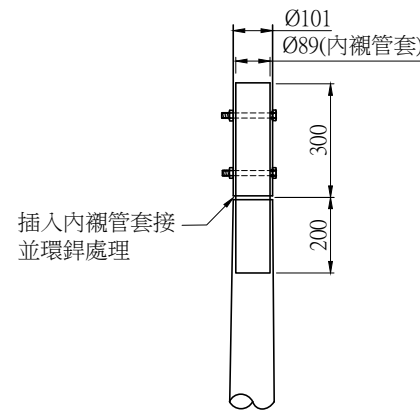
燈柱頂部插管詳圖 NTS Unit:mm
