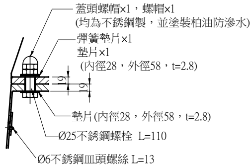
H型基座A-A 詳圖 A1 (2:1) A3 (1:1) Unit:mm
