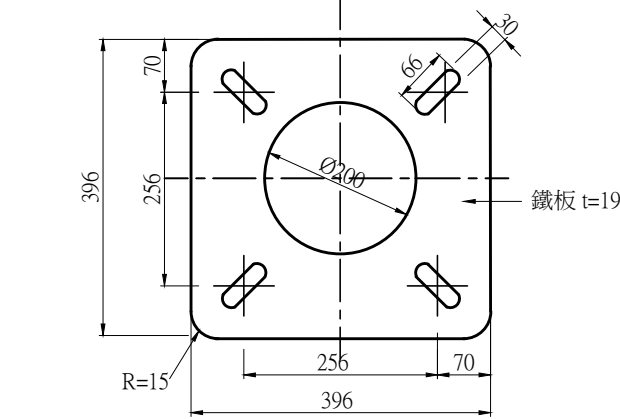
H型基座底部鐵板詳圖 A1 (1:5) A3 (1:10) Unit:mm
