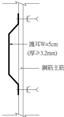
護耳(SPACER)詳圖
