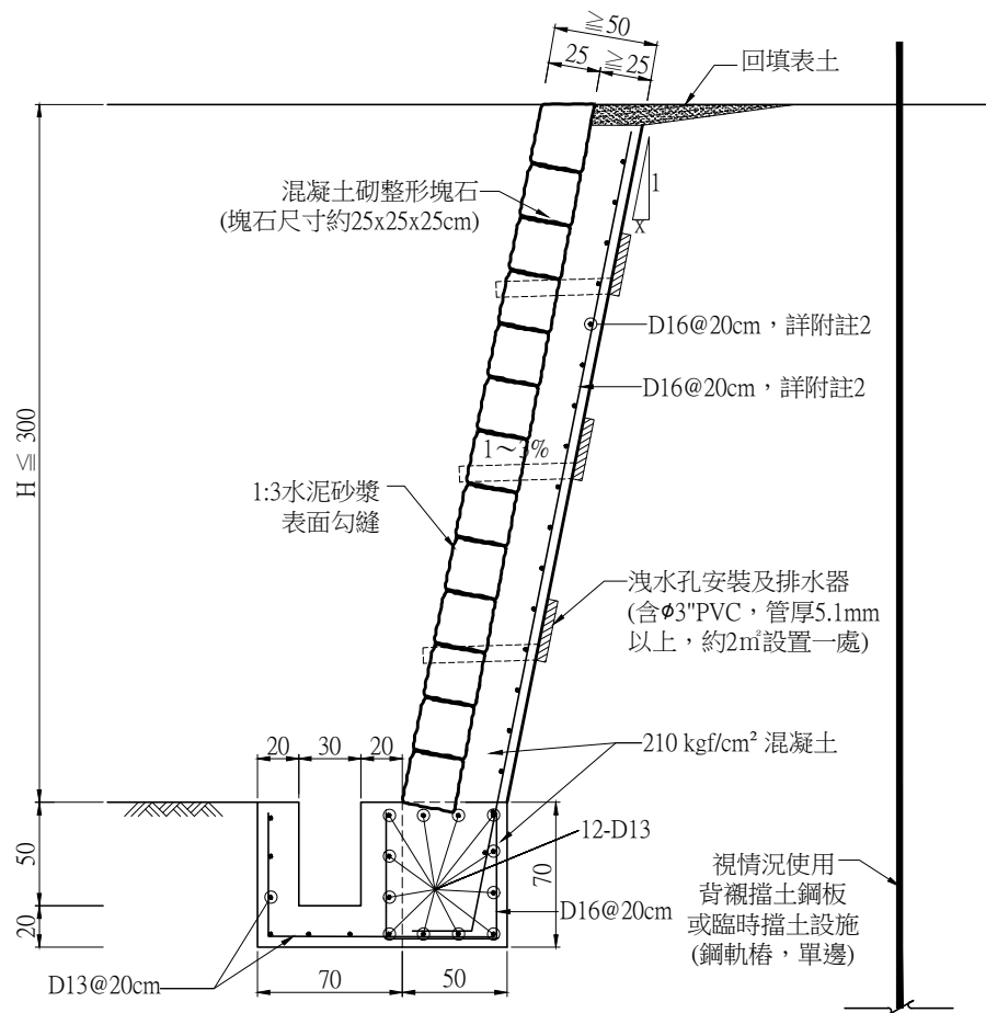
漿砌整形塊石駁坎(A型)詳圖 NTS Unit:cm
