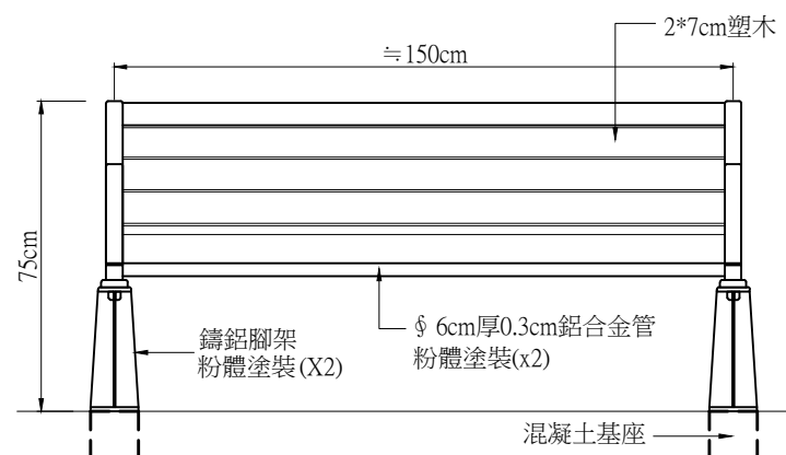
立面圖
