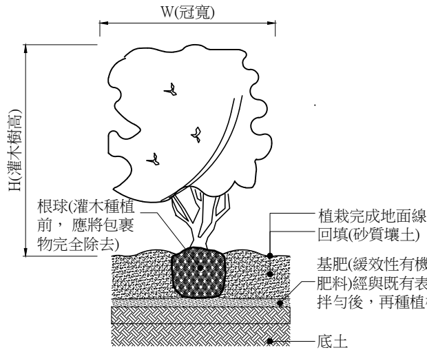
灌木栽植(單株)示意圖 NTS
