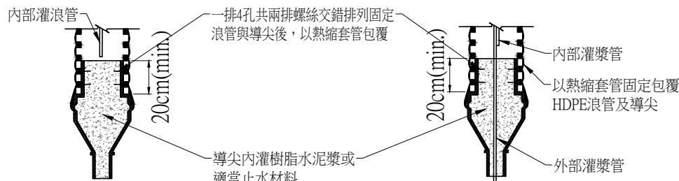
閉口導尖處理詳圖
