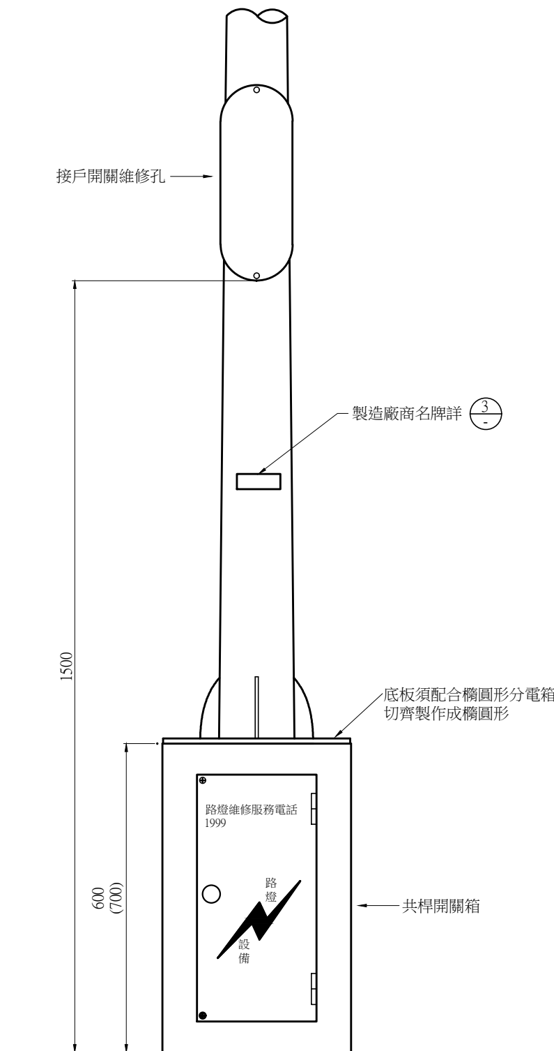
接戶開關維修孔示意圖 NTS Unit:mm
