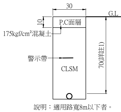
說明：適用路寬8m以下者。 DUCT C1(機械) DUCT C2(人工) NTS Unit:cm
