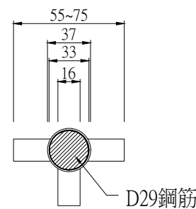
土釘中心固定器剖面示意圖 NTS Unit:mm
