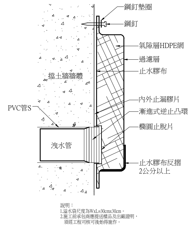
T型排水器裝設示意圖 NTS Unit:cm
