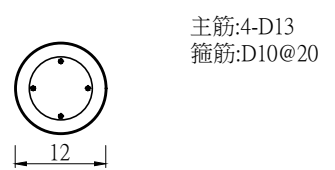
Ø12cm 仿松欄杆配筋 A1 (1:5) A3 (1:10) Unit:cm
