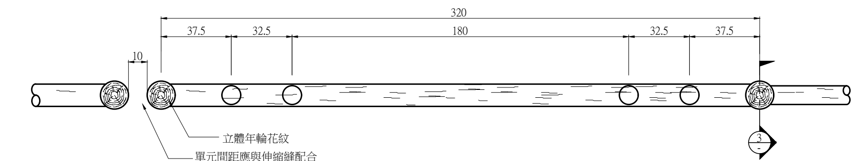
仿松欄杆(TYPE II)平面圖 A1 (1:10) A3 (1:20) Unit:cm
