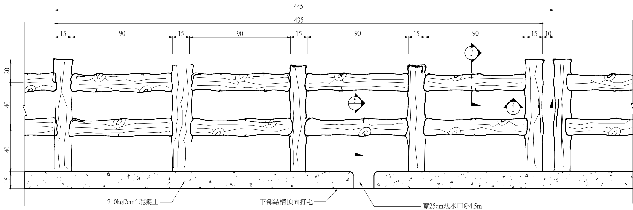
仿松欄杆(TYPE I)詳圖
