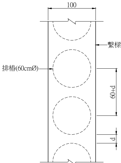
排樁擋土牆平面示意圖 (樁徑Ø=60cm)
