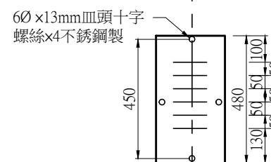
燈柱頂部插管詳圖 A1 (1:10) A3 (1:20) Unit:mm 1 -
