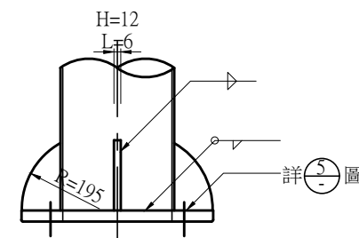
燈桿底板詳圖 NTS Unit:mm 3 -
