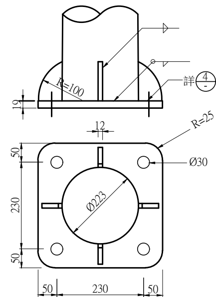
燈桿底板詳圖 NTS Unit:mm
