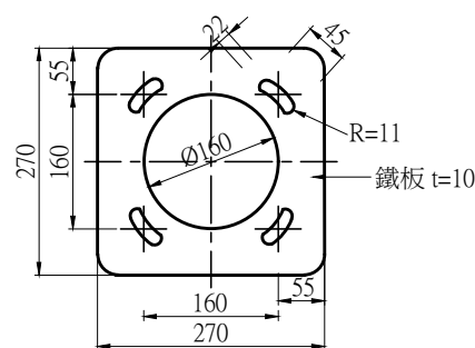
L 型基座底部鐵板詳圖 A1 (1:5) A3 (1:10) Unit:mm
