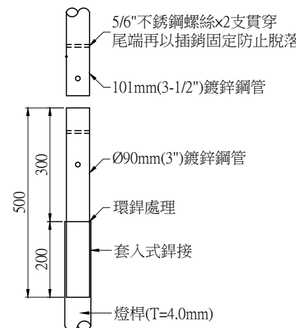
燈桿與支架套管銜接圖 NTS Unit:mm
