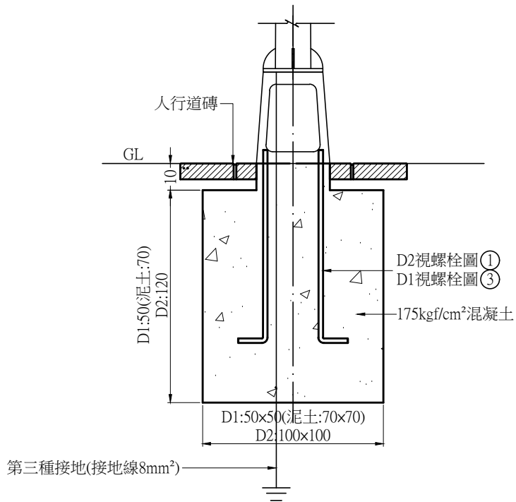
基座式(B)燈桿基礎(設於人行道) NTS Unit:cm
