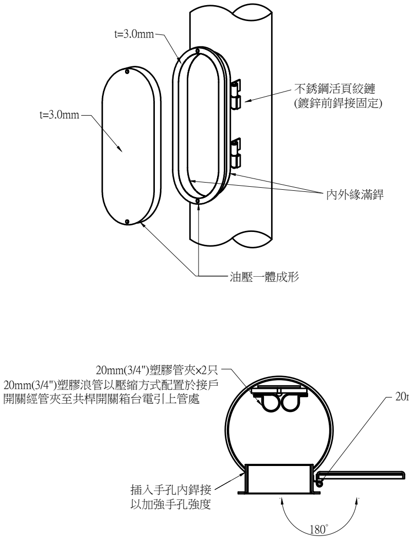
接戶開關維修孔示意圖 NTS Unit:mm
