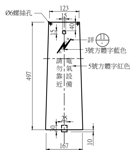
L 型基座門蓋詳圖 A1 (1:5) A3 (1:10) Unit:mm
