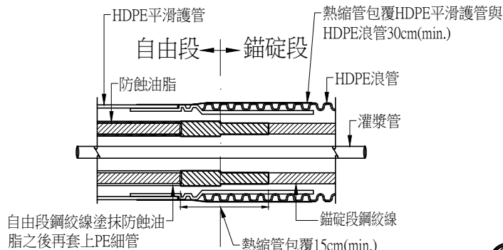
自由段平滑護管與錨碇段浪管連接處示意圖(入鋼絞線困難時)
