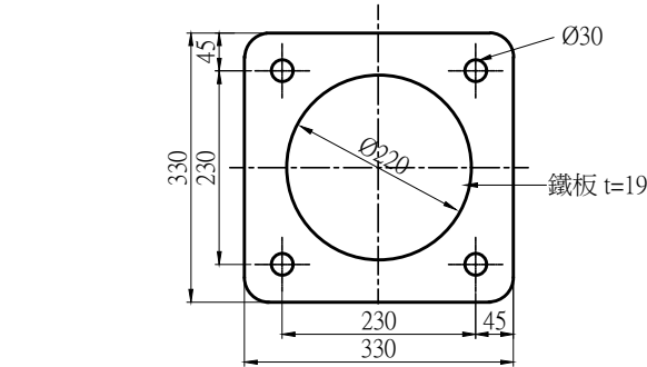
H型基座頂部鐵板詳圖 A1 (1:5) A3 (1:10) Unit:mm
