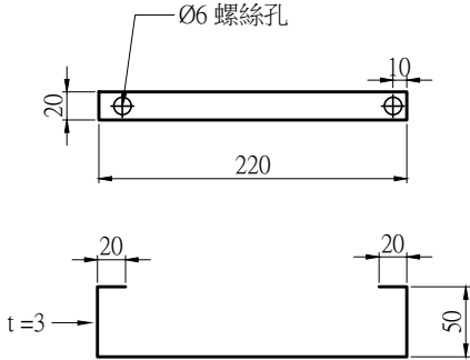
H型基座底部鐵板詳圖 A1 (1:3) A3 (1:6) Unit:mm
