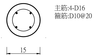
Ø15cm 仿松欄杆配筋 A1 (1:5) A3 (1:10) Unit:cm
