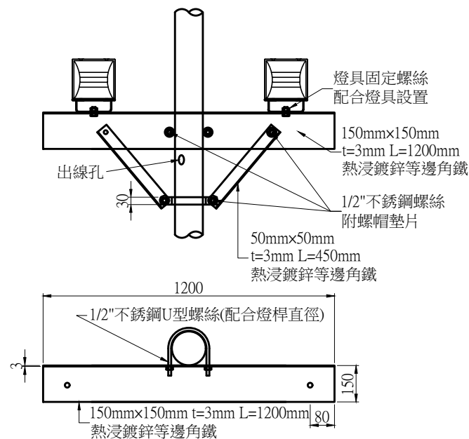
投光燈架俯視圖
