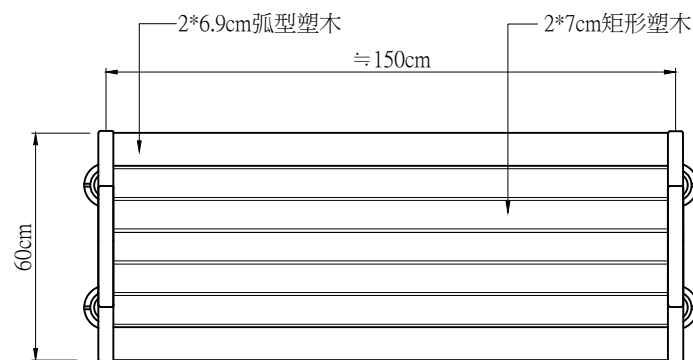
平面圖
