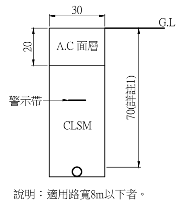
說明：適用路寬8m以下者。 DUCT A1(AC,機械) DUCT A3(AC,人工) NTS Unit:cm
