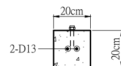
正立面圖
