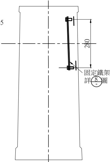
H型基座D-D 剖面圖 NTS Unit:mm
