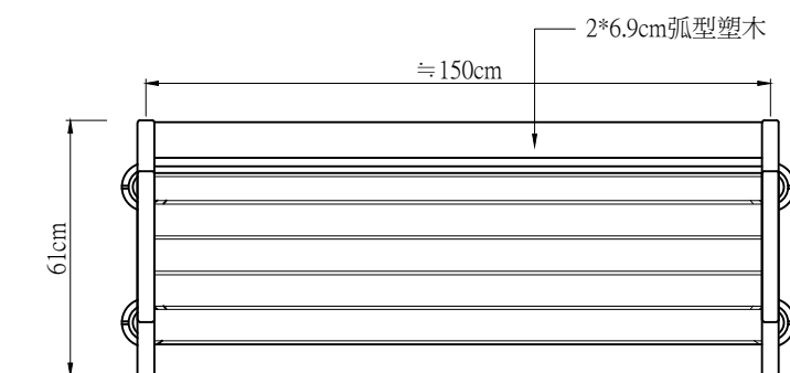
平面圖
