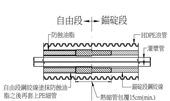
自由段與錨碇段全浪管連接處示意圖
