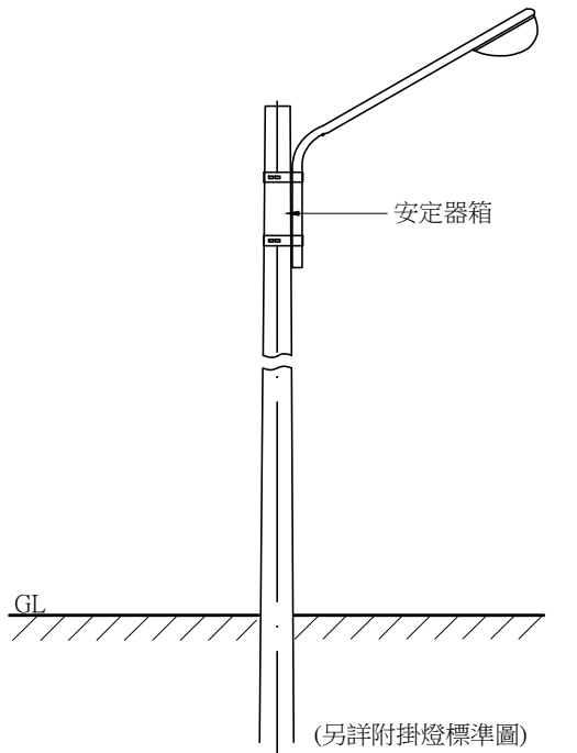
路燈安裝示意圖 NTS Unit:mm =5
