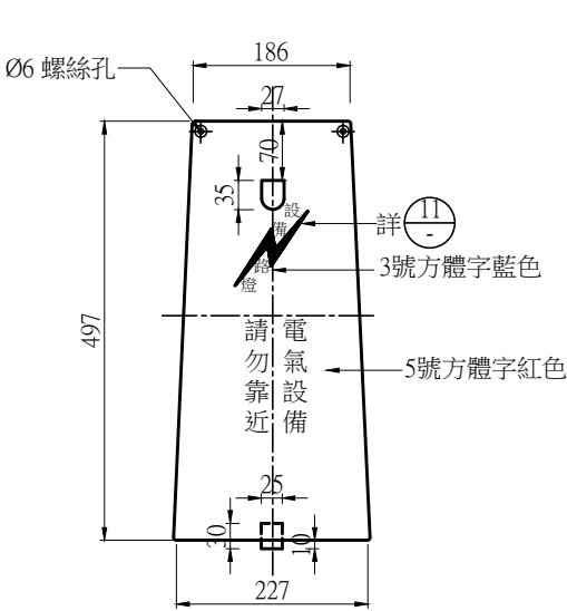
H型基座門穴詳圖 A1 (1:5) A3 (1:10) Unit:mm
