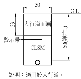
說明：適用於人行道。 DUCT E1(機械) DUCT E2(人工) NTS Unit:cm
