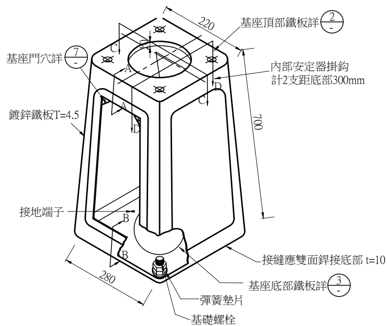
L 型基座式分電箱詳細圖 NTS Unit:mm
