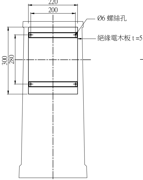
H型基座C-C 剖面圖 NTS Unit:mm
