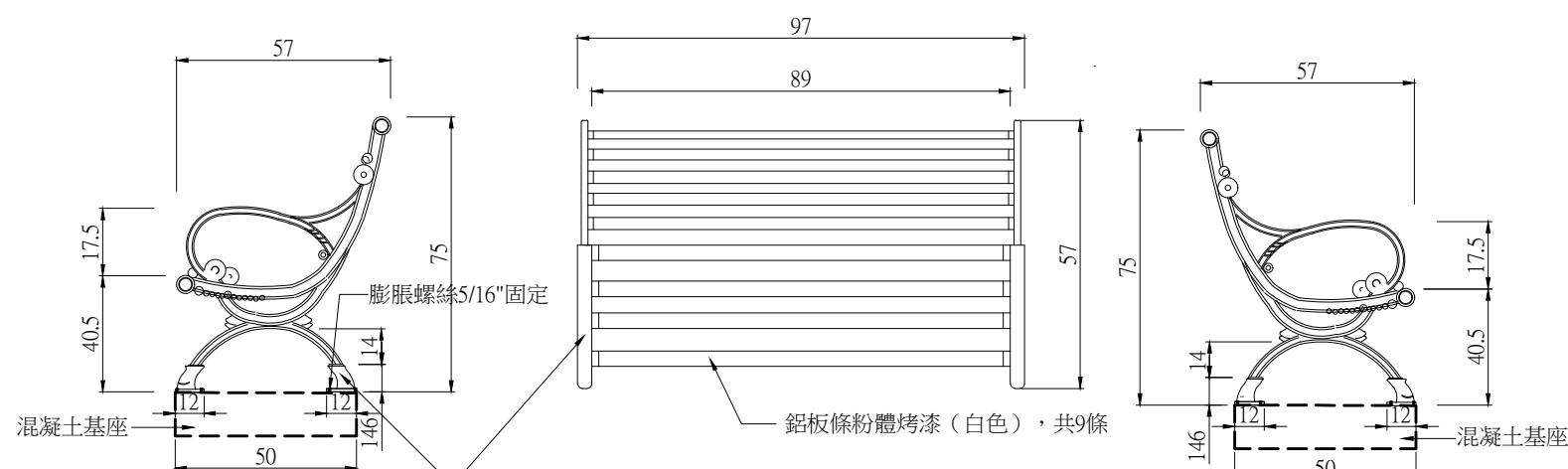
側向立面圖（右）
