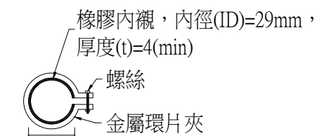
金屬環片夾詳圖 NTS Unit:mm
