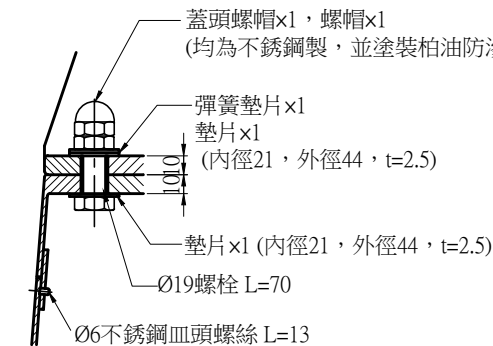
L型基座頂板剖面圖
