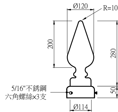
鑄鋁合金裝飾頂座 NTS Unit:mm
