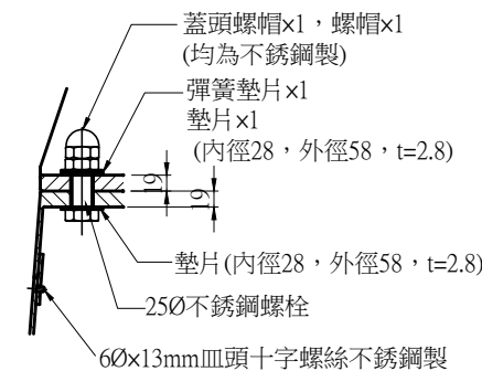
底板、H型基座接合詳圖 NTS Unit:mm
