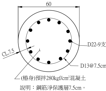
Ø60cm排樁配筋詳圖
