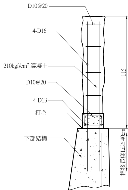
剖面圖
