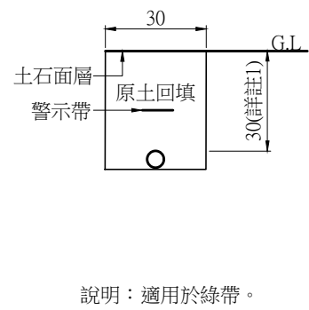
說明：適用於綠帶。 DUCT B3(機械) DUCT B4(人工) NTS Unit:cm
