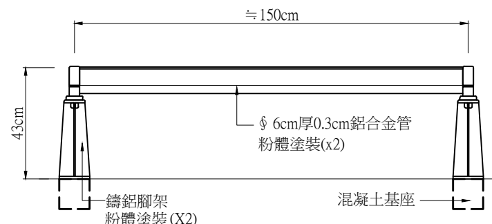
立面圖
