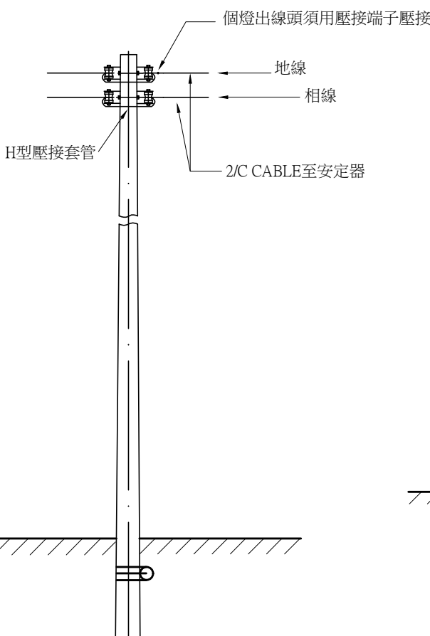
安裝圖 C NTS Unit:mm =4
