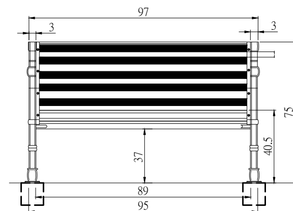
正立面圖
