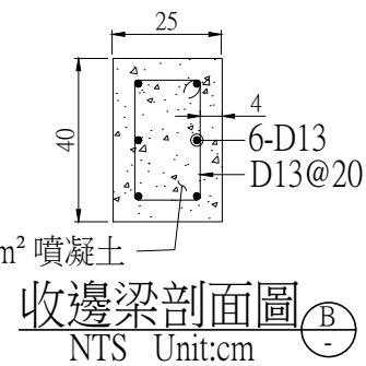
型框剖面圖 NTS Unit:cm
