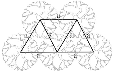
灌木及地被栽植(等三角定植)平面配置圖 NTS
