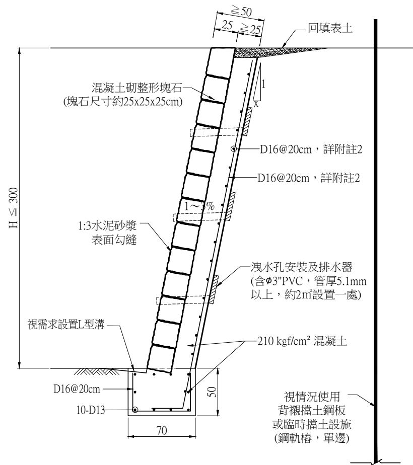
漿砌整形塊石駁坎(B型)詳圖 NTS Unit:cm
