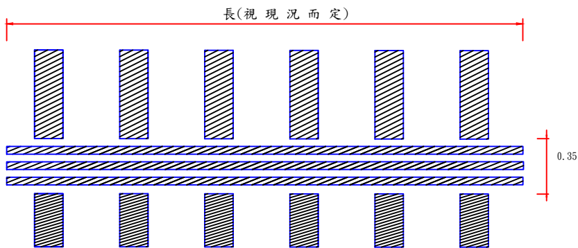
⑨c) 視覺功能障礙引導標線 §185 §186 (刨除長x0.35；長x0.15x3)(劃設2至3次，厚度0.4至0.6公分)
