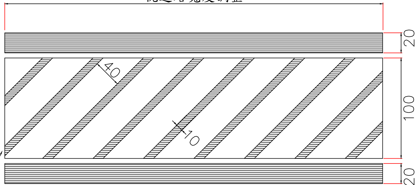
減速丘鋪面劃設黃色斜紋標線
