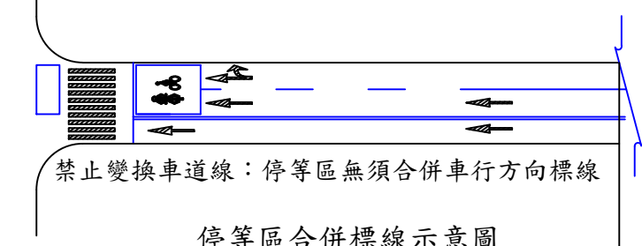
停等區合併標線示意圖
