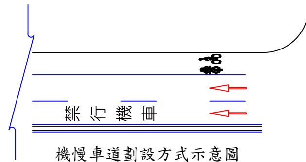
機慢車停等區劃設方式示意圖
