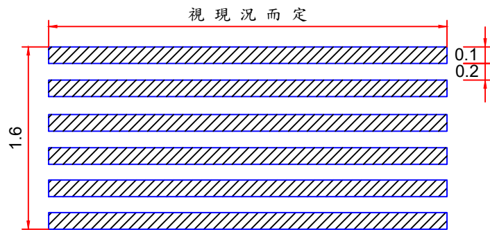
⑪ 減速標線 §159 (長x0.6x次數) 範例: ⑪ 1 表示標線劃1次，厚度0.2cm ⑪ 2 表示標線劃2次，厚度0.4cm ⑪ 3 表示標線劃3次，厚度0.6cm
