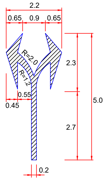
31 分岔箭頭(3) §188 (數量:5m 2 ) 註:限用20cm漏斗。
