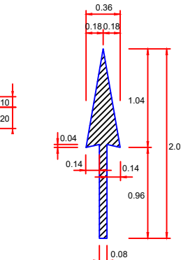
36-12 自行車穿越道線之直線箭頭 (數量:0.5m)
