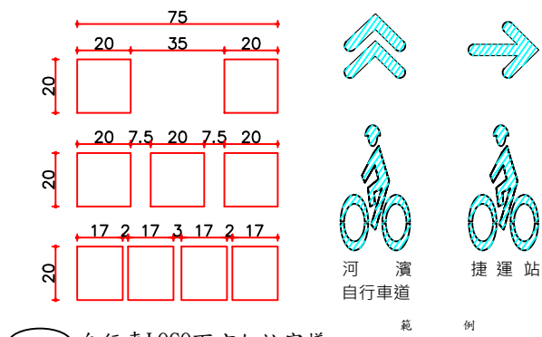
36-10 自行車LOGO下方加註字樣 (字樣以設計圖為準)
