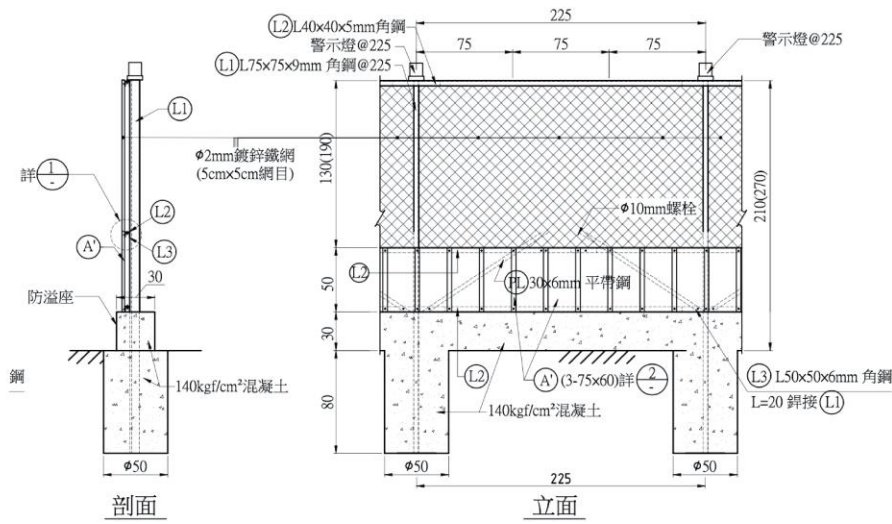
半阻隔式固定圍籬(2.1m及2.7m)
