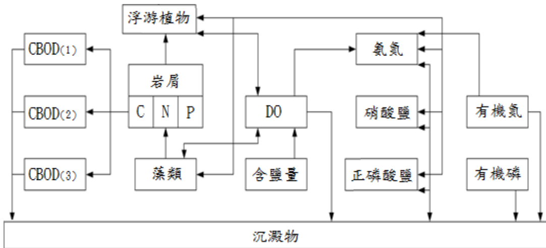
圖 1 EUTRO 模組基本架構
