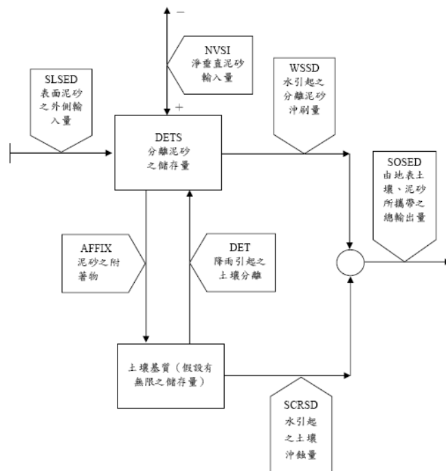
圖9 SEDMNT 副程式之演算流程
