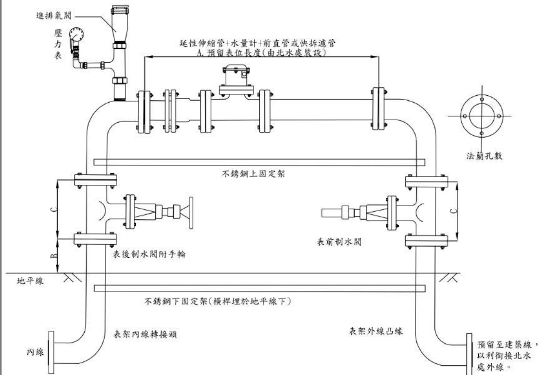
地上式大表表位架示意圖
