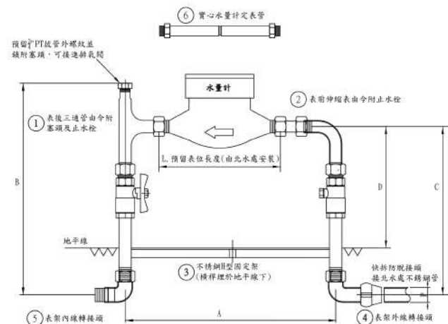
地上式中、小表表位架示意圖
