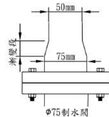
圖a. Ø75x50mm縮管
