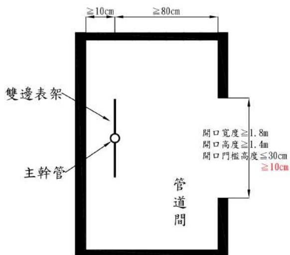
俯視圖
