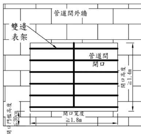
管道間開口正視圖
