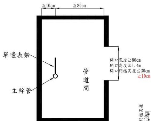
俯視圖
