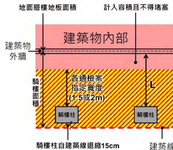
平面圖
