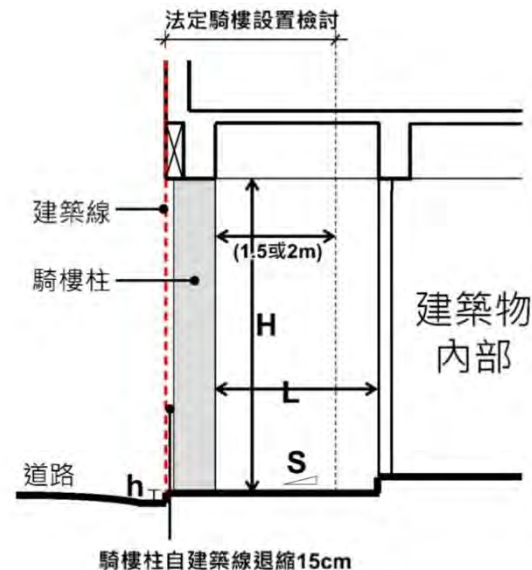
剖面圖
