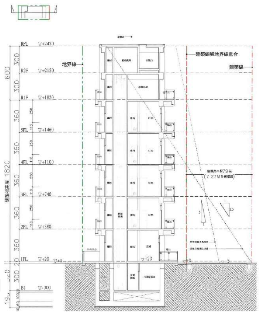
橫向剖面圖 S:1/150
