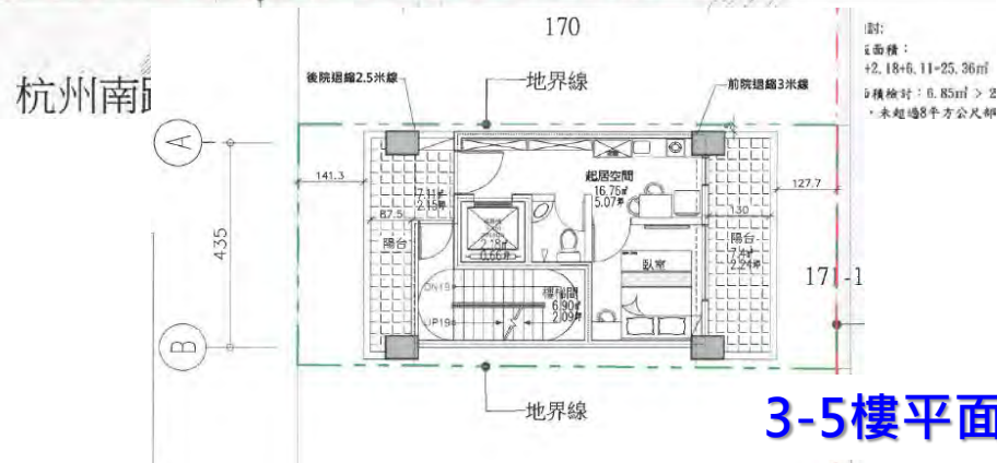
1樓平面圖
