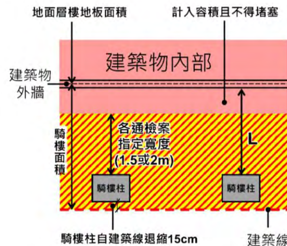
平面圖
