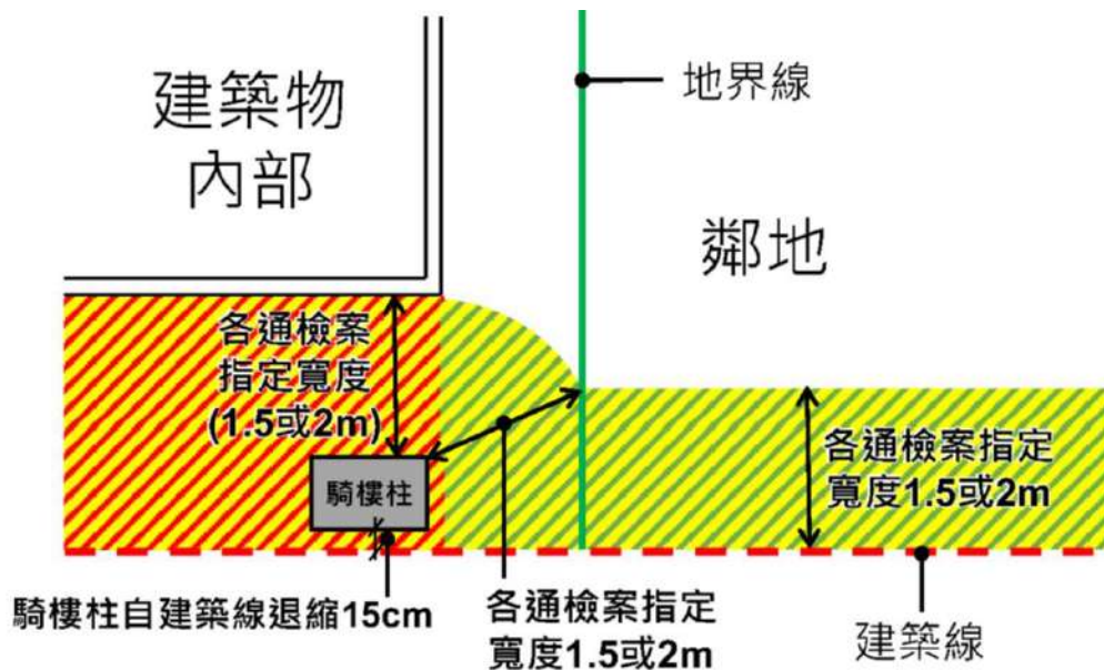
平面圖
