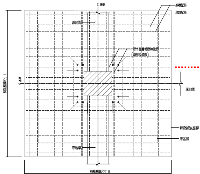
RC擴柱新設補強基礎平面圖
