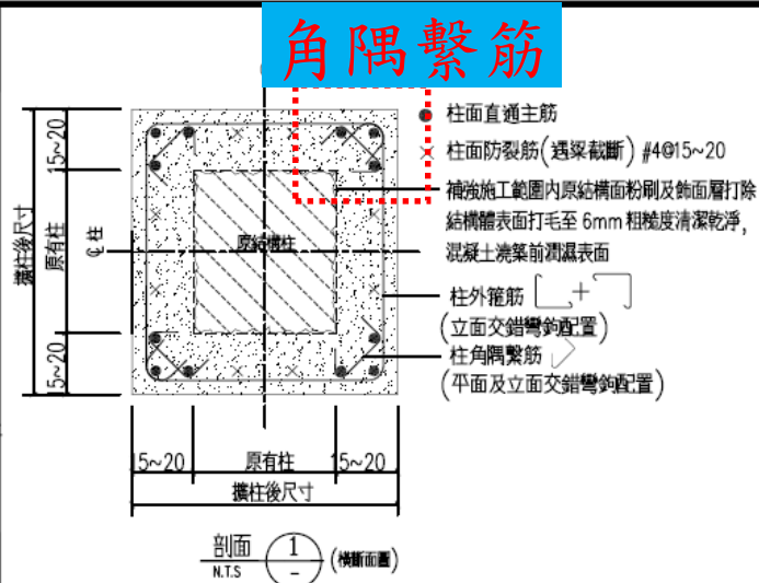
RC擴柱補強斷面詳圖(方案一)
