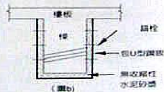
RC梁強度不足時可以鋼板來補強
