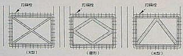
建築師需要良好通風採光時，可以採用鋼樑加斜撐來做補強
