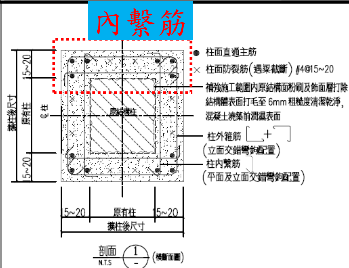
RC擴柱補強斷面詳圖(方案二)
