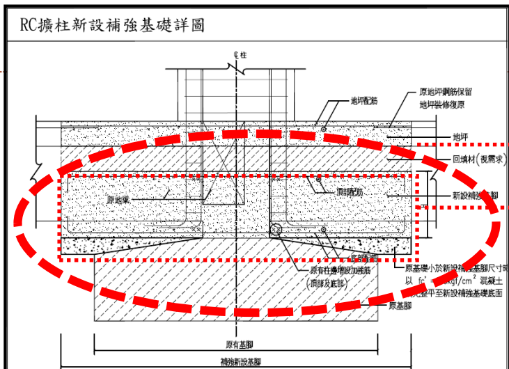
RC擴柱新設補強基礎剖面圖
