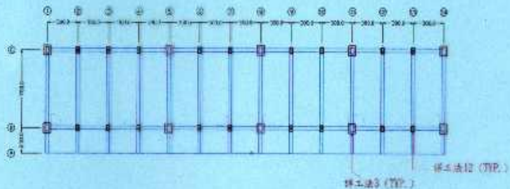
長流國小公園(一)一層結構佈置平面圖 1:100
