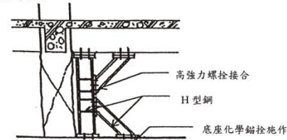
3. K型斜撐臨時支撐
