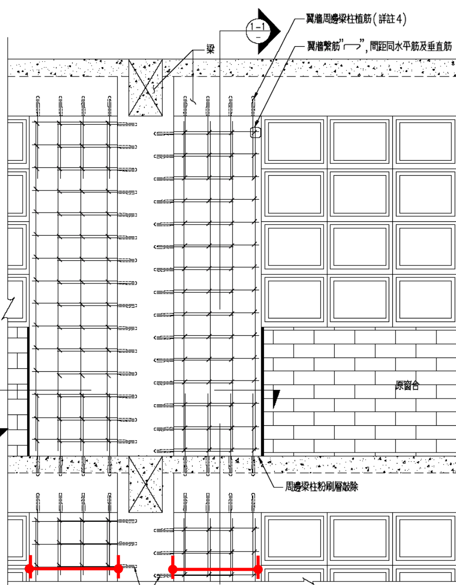
1 翼牆補強立面詳圖 S=N. T.S.
