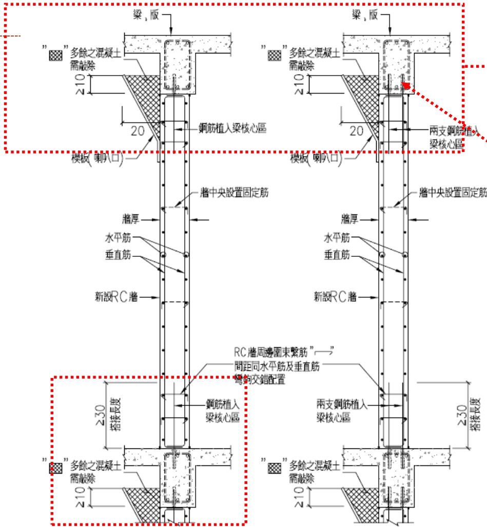
1-1 a 新增 RC 牆立剖面詳圖(方案一) S=N.T.S.
