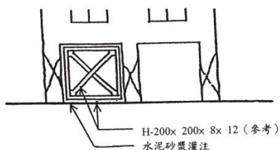
2. 鋼框鋼骨斜撐臨時支撐
