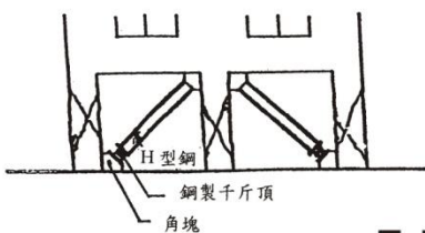
1. H型鋼斜撐臨時支撐
