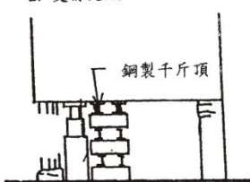
2. 支撐完成，更換主筋
