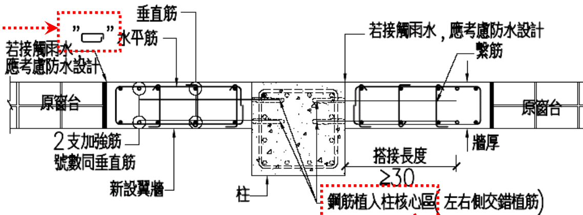
新增 RC 翼牆平剖面詳圖(方案一)
