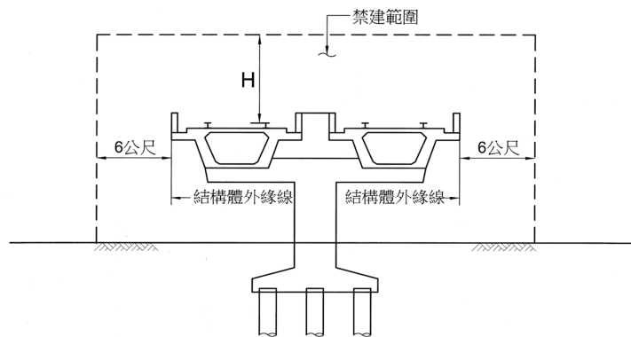
示意圖一 高架段路線禁建範圍圖
