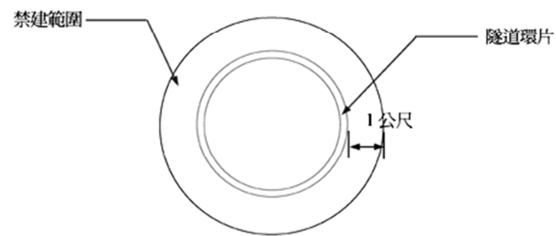
示意圖四 潛盾隧道禁建範圍圖
