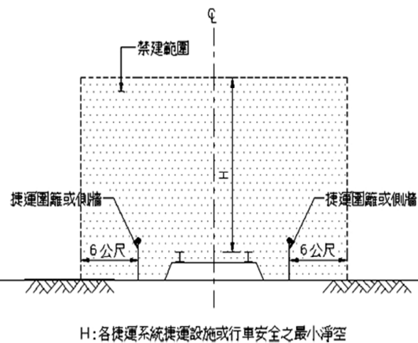
示意圖三 地面段路線禁建範圍圖
