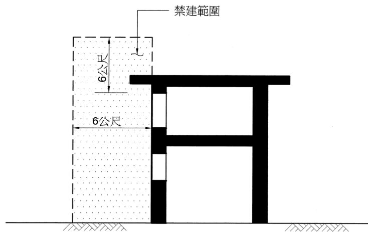
示意圖七 通風井禁建範圍圖
