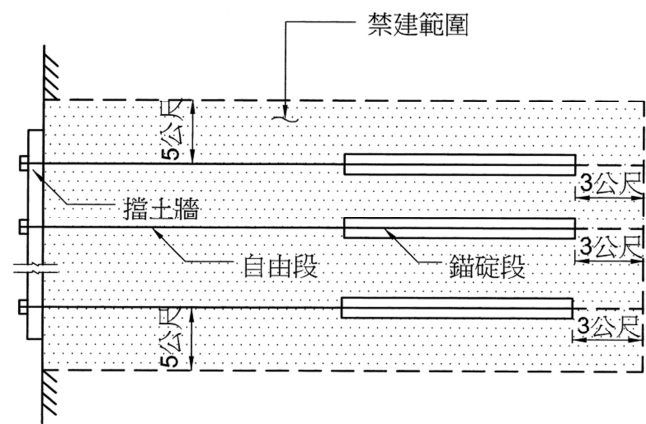
示意圖六之二 錨固邊坡禁建範圍圖（平面）
