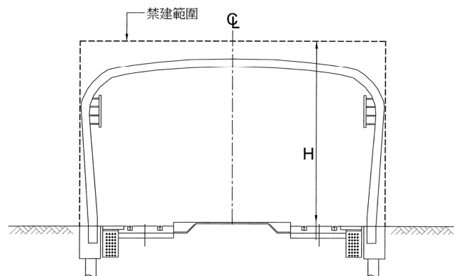
示意圖八之二 非完全獨立專用路權之平面段禁建範圍(架空線)
