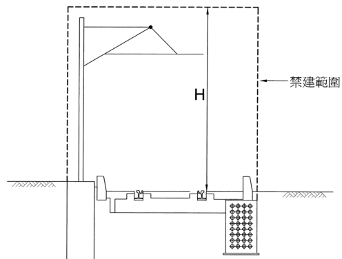
示意圖八之二 非完全獨立專用路權之平面段禁建範圍(架空線)
