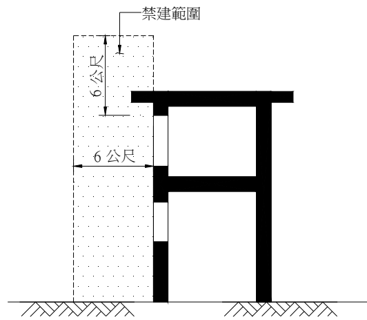
示意圖七 通風井禁建範圍圖
