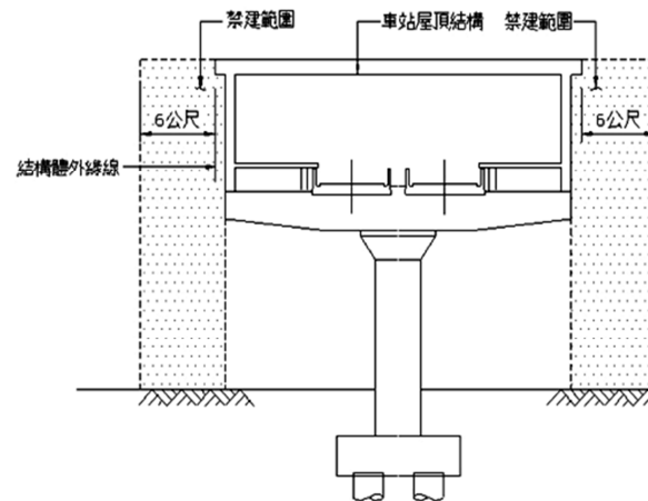
示意圖二 高架段車站禁建範圍圖
