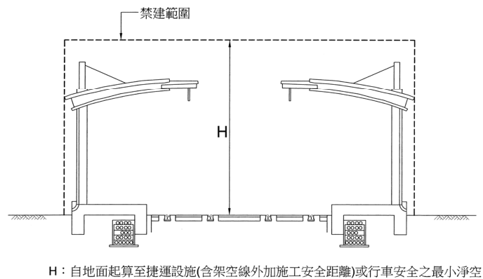
示意圖九之二 非完全獨立專用路權之平面車站段禁 建範圍(車站型式二)
