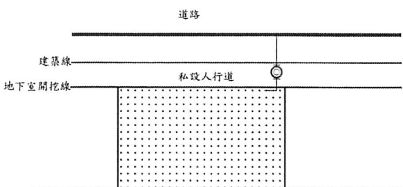
1-4 建築物表位設於私設人行道
