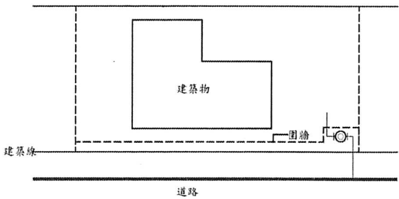
1-3 洋房式建築表位設於圍牆外側牆邊
