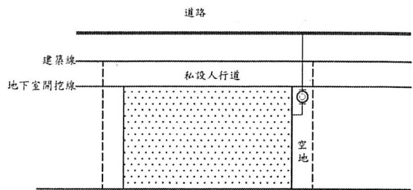
1-5 建築物有私設人行道路，且兩旁有空地者，表位退縮至私設人行道後之空地，惟考量日後外線之維護，應經申請人之同意。
